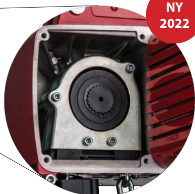
Kædestyr er let tilgængelig for vedligeholdelse / Chain guide easily accessible for maintenance purposes
